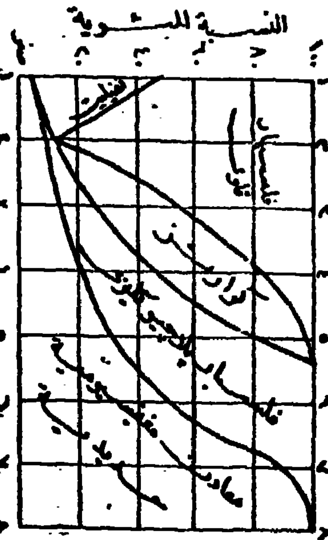
( شكل رقم ٣ ) التكوين المعدني العام للصخور النارية العادية
